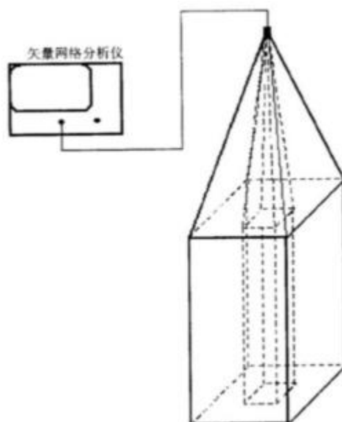
图 5 低频同轴反射法测试布置示意图
