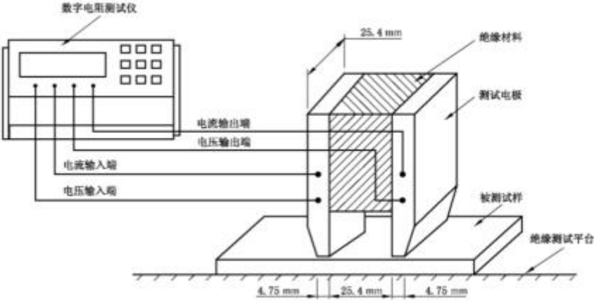
图 2 表面电阻测试布置图
