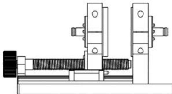
图 8 30MHz~3GHz 法兰同轴装置
