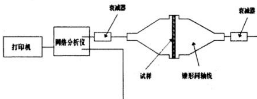
图 9 法兰同轴装置测试法布置图
