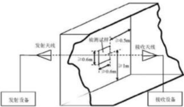
图 4 屏蔽室测试法布置图
