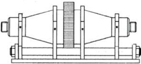
图 7 30MHz~1.5GHz 法兰同轴装置
