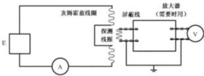
图 3 低频磁场测试原理图
