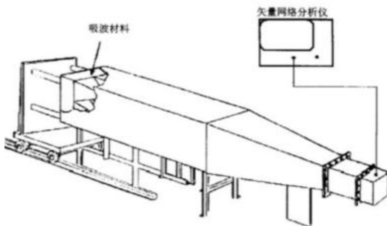
图 6 波导法测试布置示意图
