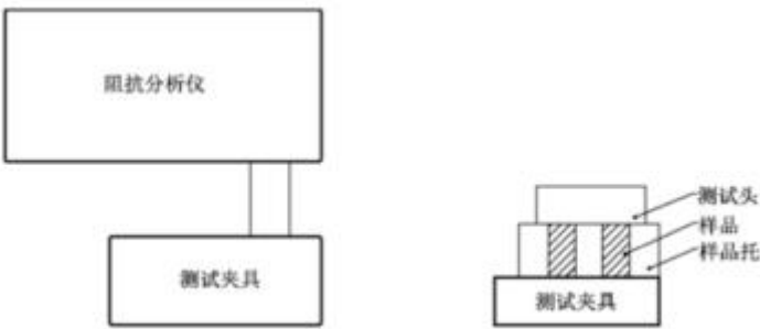
图 1 磁导率测试布置示意图
