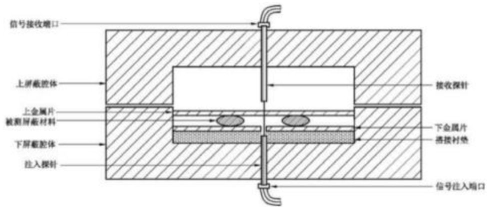
图 10 射频导电性能测试夹具示意图
